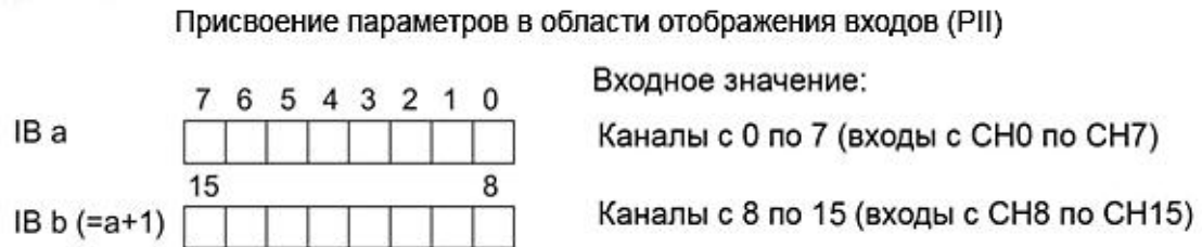
Рисунок 4-1 Пространство адресов для конфигурации 16-ти канального модуля DI 16x230V AC BA
