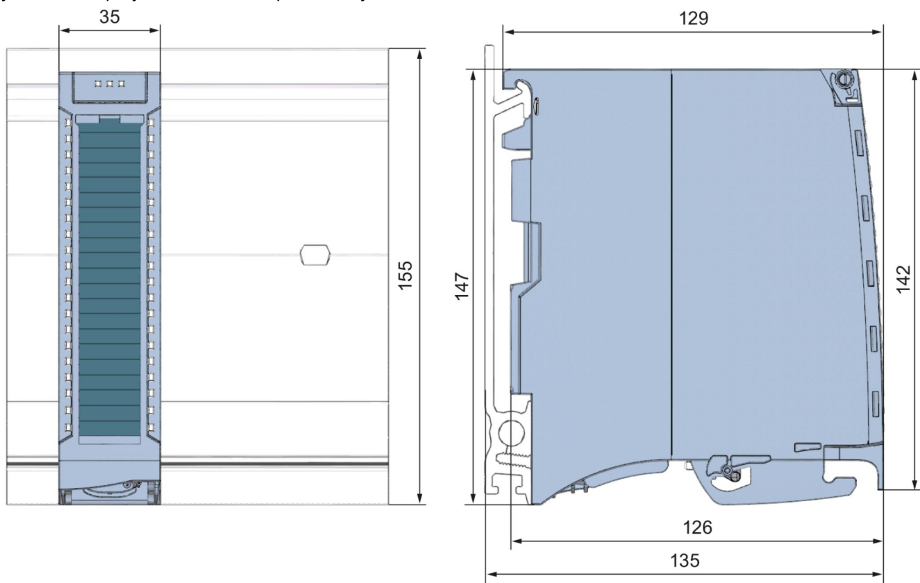
Рисунок А-1 Габаритный чертеж модуля DI 16x230V AC BA
