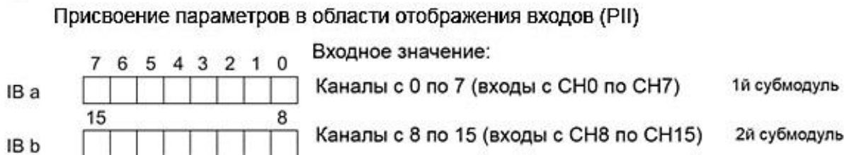
Рисунок 4-2 Пространство адресов для конфигурации модуля в режиме 2x канального входа DI 16x230V AC BA S
