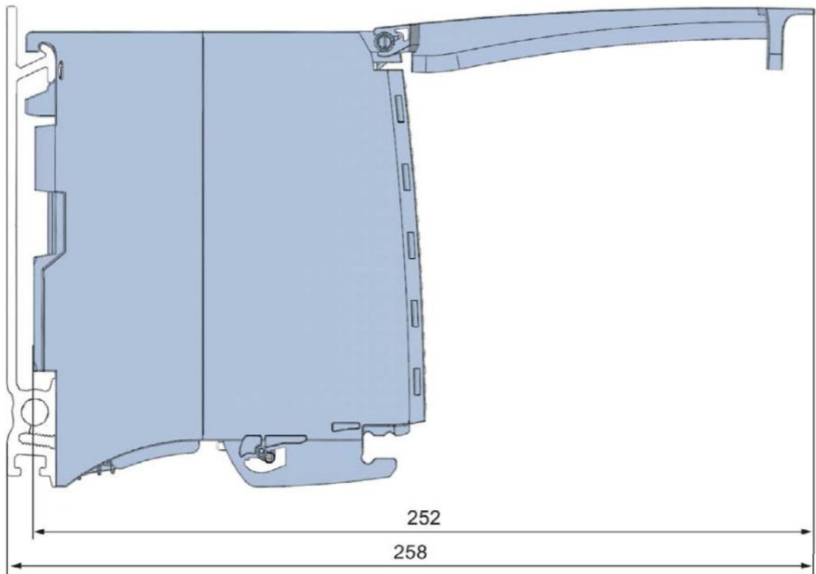
Рисунок А-2 Габаритный чертеж модуля DI 16x230V AC BA вид сбоку, с открытой передней крышкой
