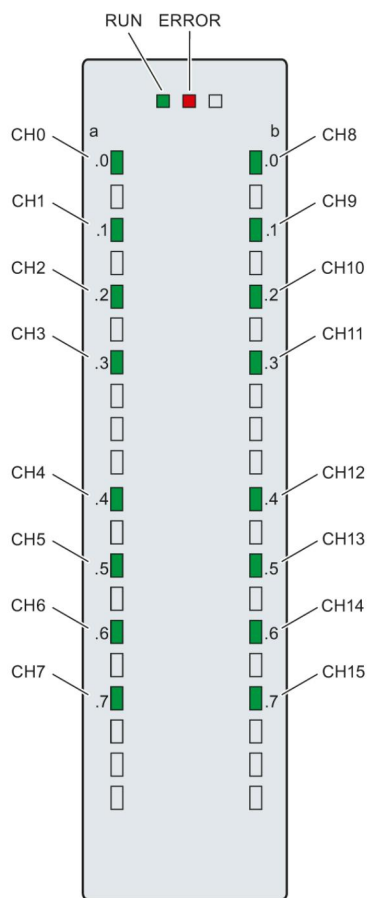
Рисунок 5-1 Светодиодные индикаторы модуля DI 16x230V AC BA
