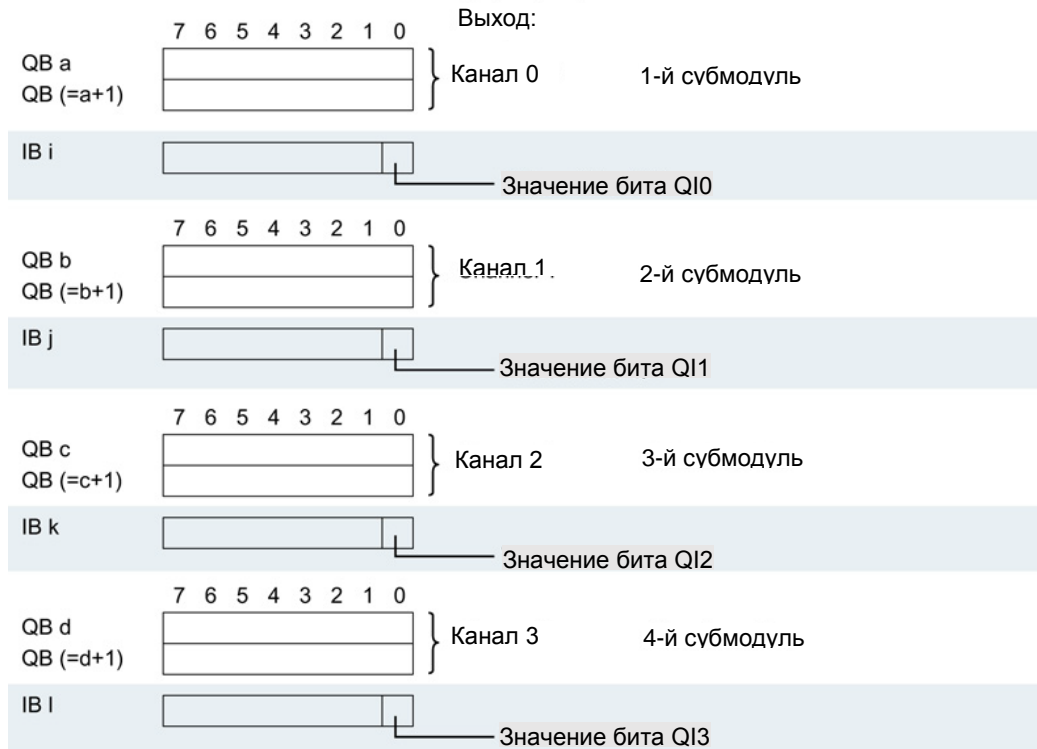
Рис. 4-2 Адресное пространство для конфигурации 4 x 1 канал модуля AQ 4xU/I ST S QI с регистрацией информации о качестве
