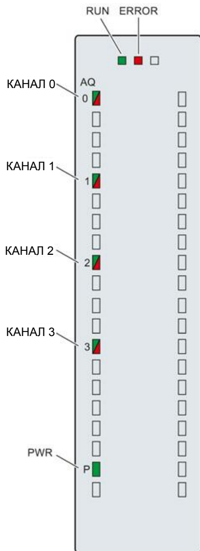
Рис 5-1 Светодиоды индикации модуля AQ 4xU/I ST
