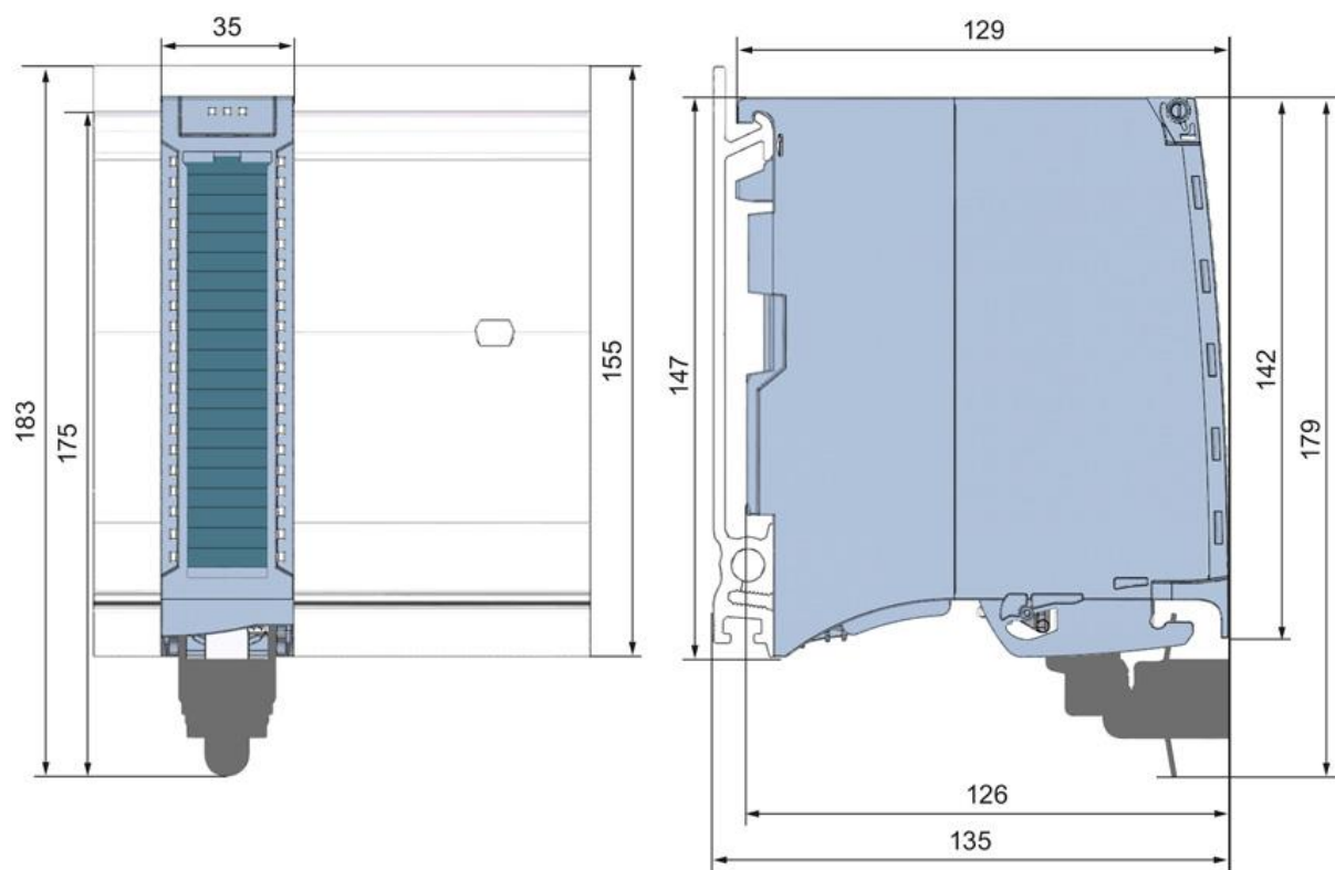
Рис. А-1 Габаритный чертеж модуля AQ 4xU/I ST
