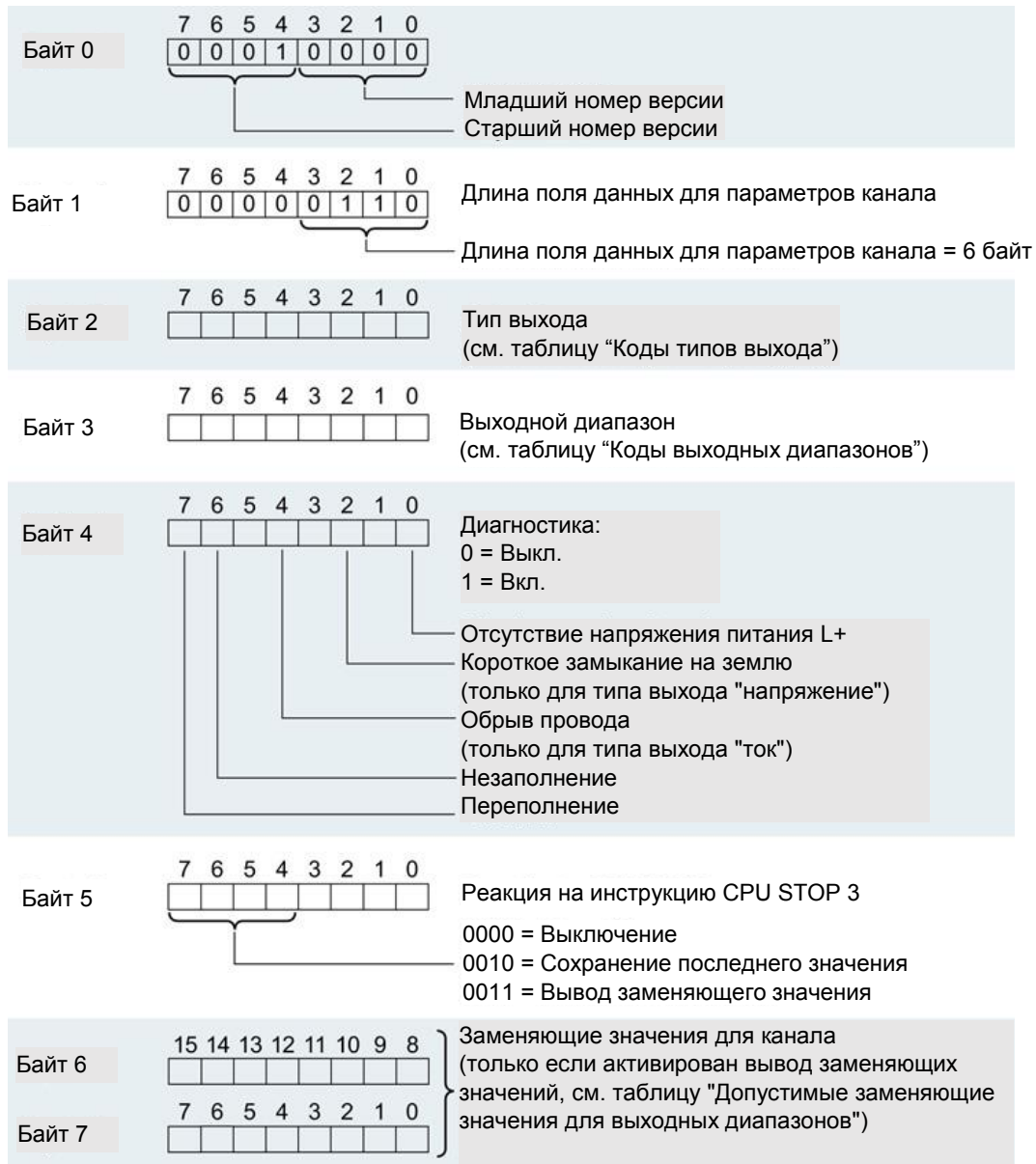
Рис. А-1 Структура записи данных 64: Байты с номерами от 0 до 7
