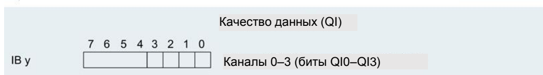
Рис. 4-1 Адресное пространство модуля AQ 4xU/I ST в конфигурации 1 x 4-каналов с регистрацией информации о качестве
