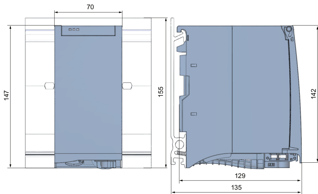
Рисунок А-1 Габаритный чертеж блока питания PS 60W 24/48/60VDC
