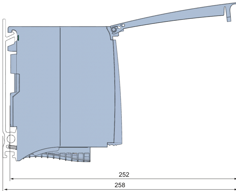
Рисунок А-2 Габаритный чертеж блока питания PS 60W 24/48/60VDC, вид сбоку с открытой передней панелью
