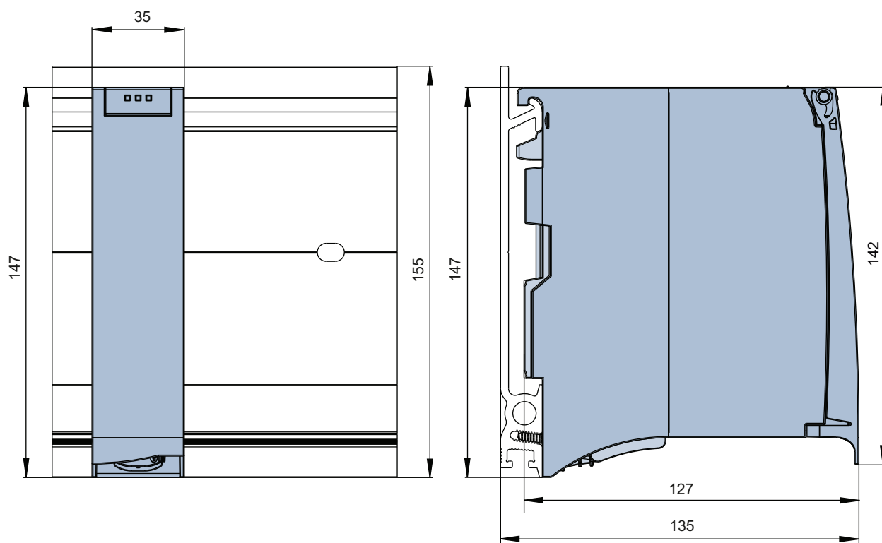
Рисунок А-1 Габаритные размеры коммуникационного модуля CM PtP RS232 BA
