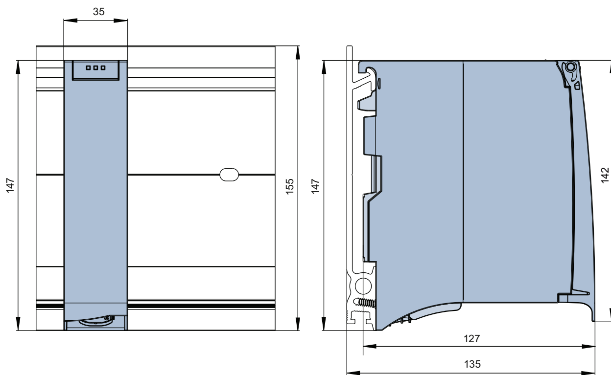
Рисунок А-1 Габаритные размеры коммуникационного модуля CM PtP RS422/485 BA
