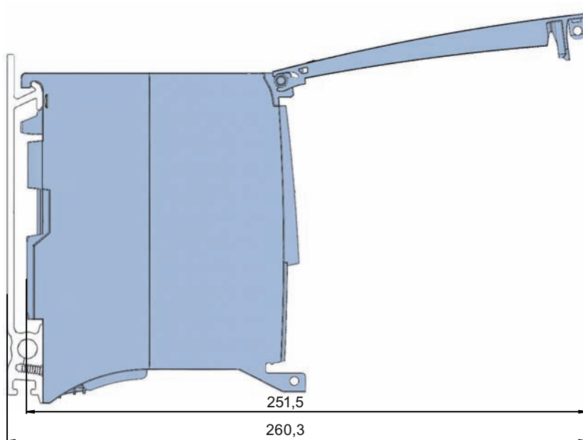
Рисунок А-2 Габаритные размеры коммуникационного модуля CM PtP RS422/485 BA с открытой передней панелью
