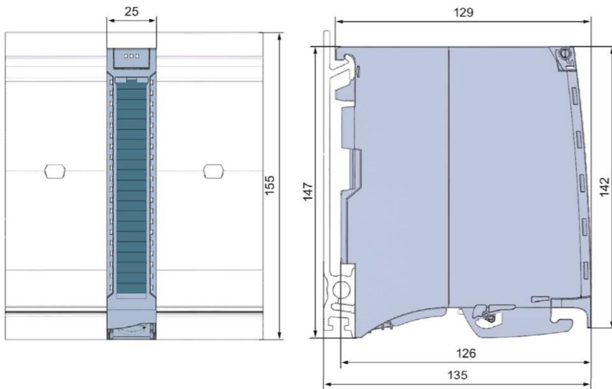
Рисунок А-1 Габаритный чертеж модуля DQ 32x24VDC/0.5A BA
