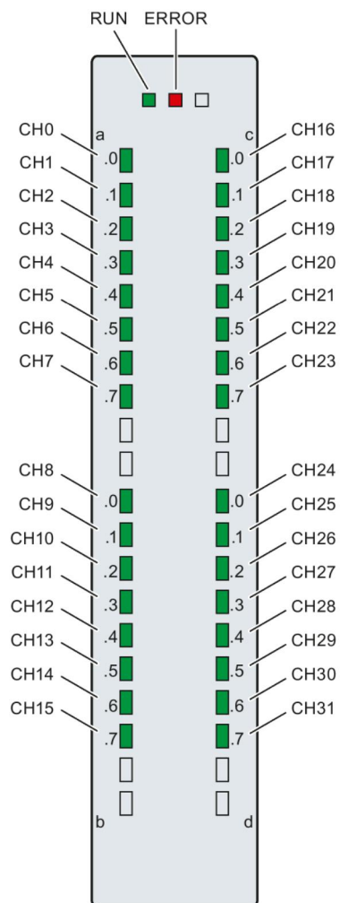
Рисунок 5-1 Светодиодные индикаторы модуля DQ 32x24VDC/0.5A BA
