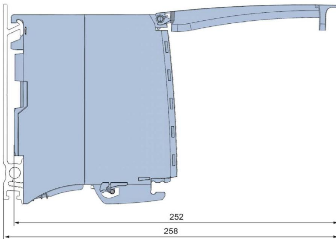
Рисунок А-2 Габаритный чертеж модуля DQ 32x24VDC/0.5A BA вид сбоку, с открытой передней крышкой
